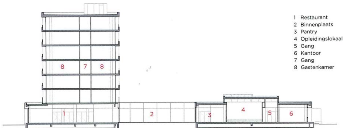
Doorsnede
